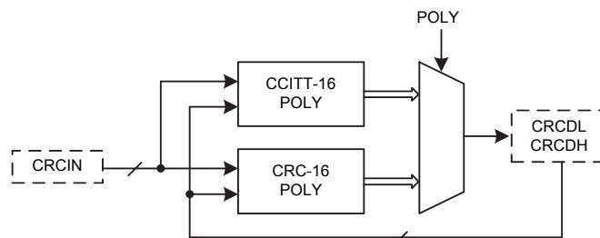
CRC 方框图
