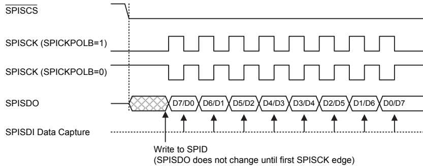
SPI 从机模式时序 – SPICKEG=0
