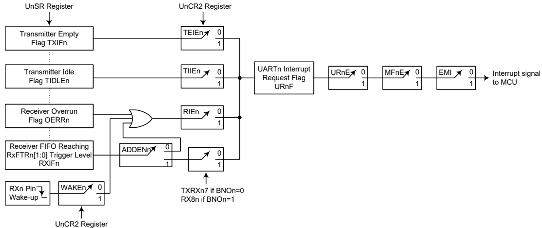
UARTn 中断框图
