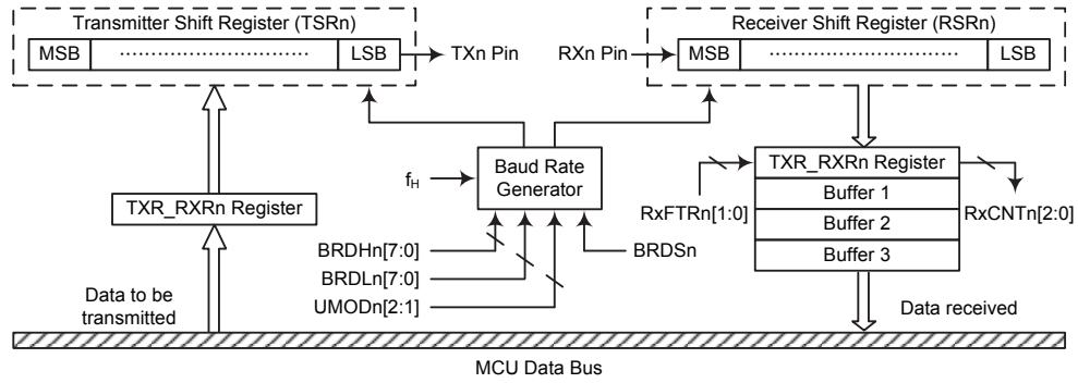
UARTn 数据传输方框图 (n=0~1)
