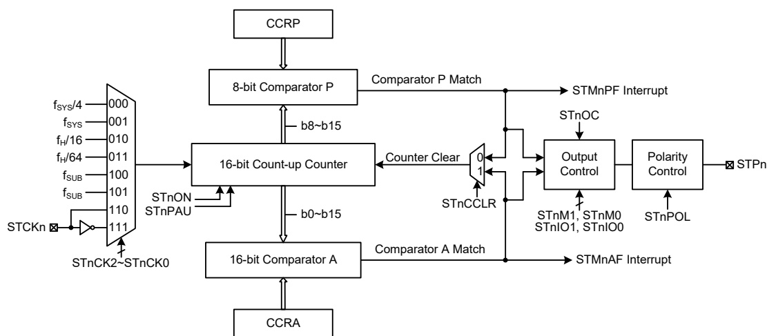
标准型 TM 方框图 (n=0~2)
