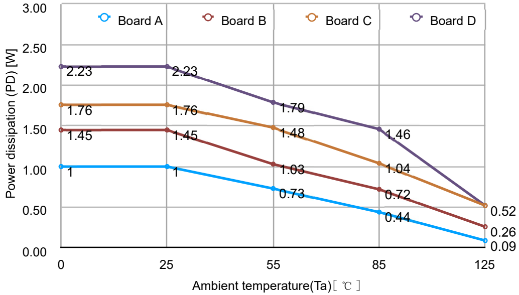
(2) 测试板 A (ESOP8)
