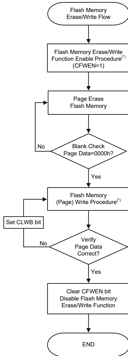
Flash 存储器擦 / 写流程
